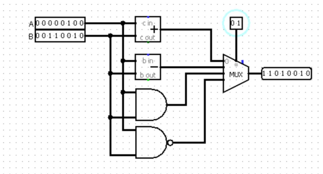
Figure 1: Cấu tạo ALU
